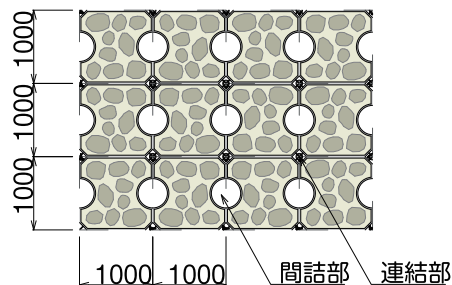
展開図
