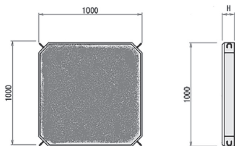
製品単体図
