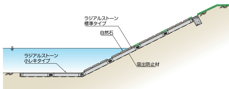
標準断面図
