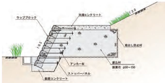
参考断面図
