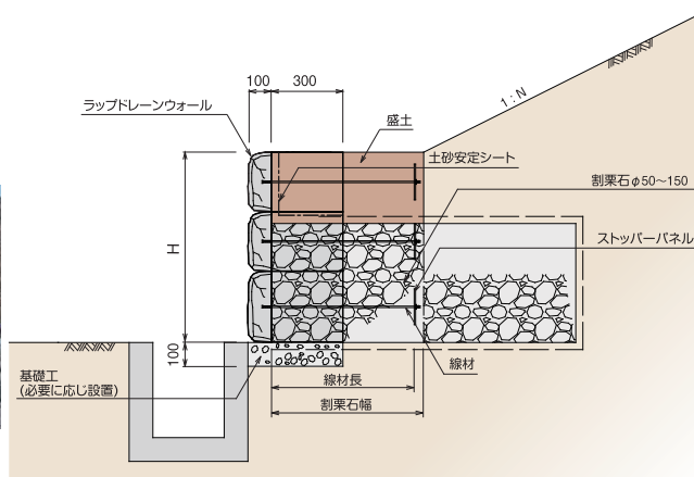
標準断面図
