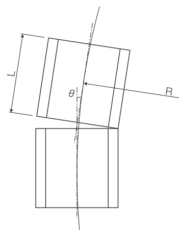
曲げ角度
