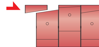
■ Kセグメント(軸方向挿入型)
