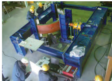
継手曲げ試験
