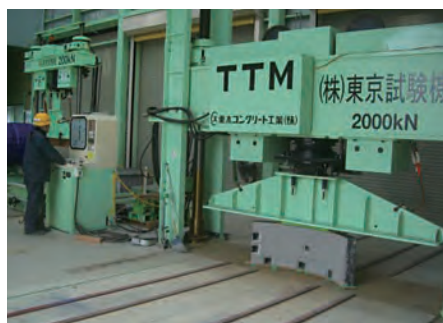
推力試験
