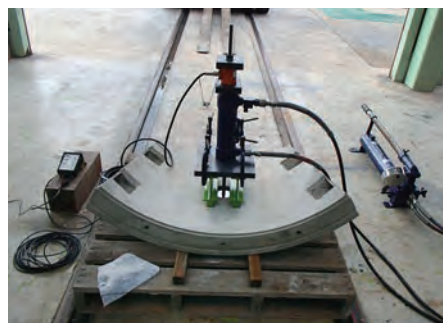
吊手引き抜き試験
