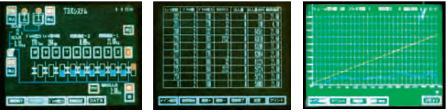
メイン画面 管ごとの管理表 推進力変移グラフ
