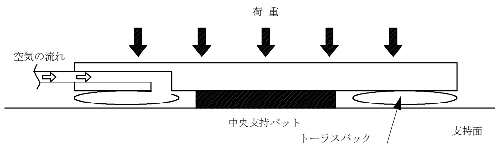
図一解 1.4.2 作動原理 (その 1)
