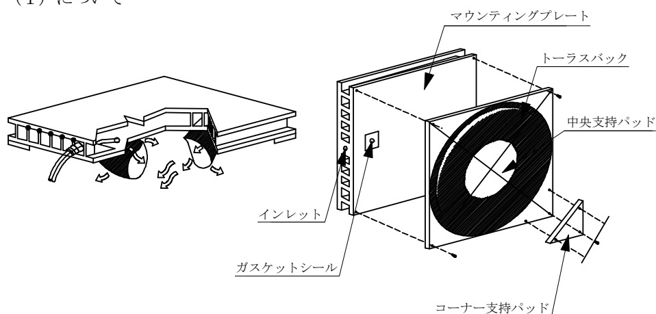
図一解 1.4.1 エアーキャスターの構造
