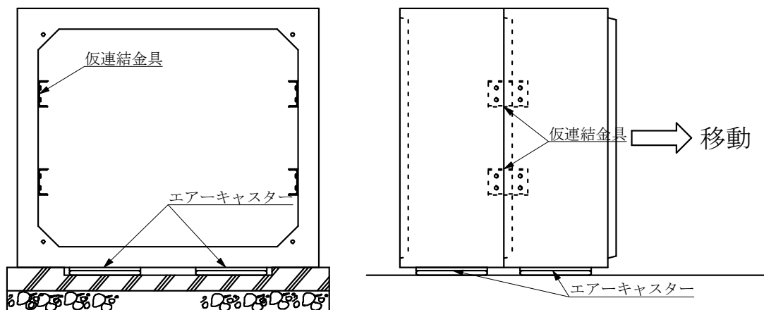
図一解 5.1.4 連結施工の例
