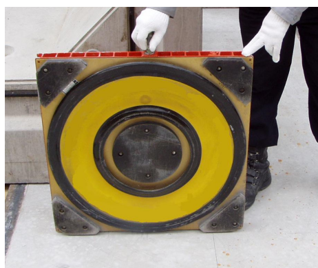
写真一解 1.4.2 滑走面 (K27UHD) の例
