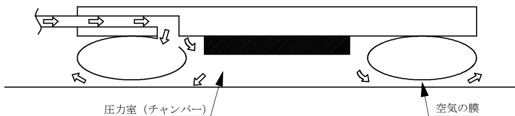
図一解 1.4.4 作動原理（その3）
